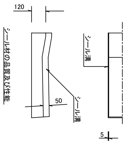
ジョイント部 詳細図 S=1/200
