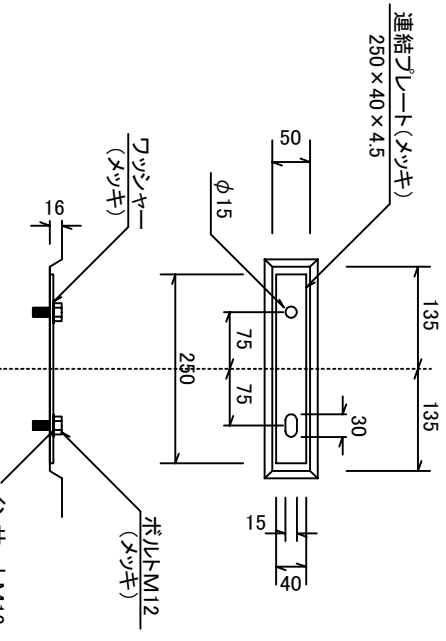
連結部詳細図 S=1/10
