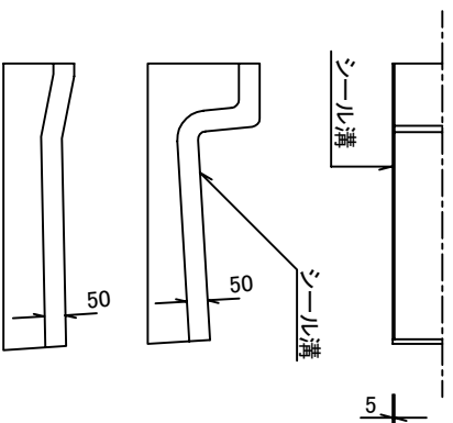
ジョイント部 詳細図 S=1/200
