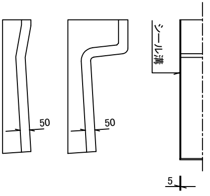
ジョイント部 詳細図 S=1/200
