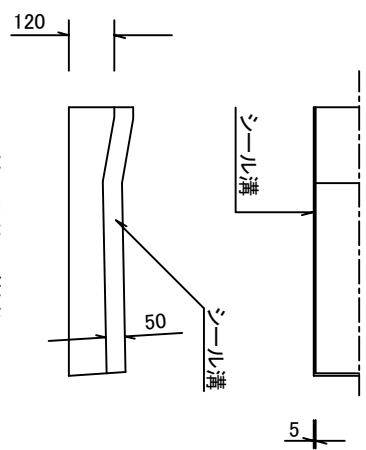
ジョイント部 詳細図 S=1/200
