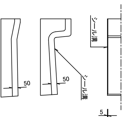
ジョイント部 詳細図 S=1/200
